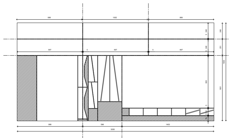
Découpe des planches de multiplis
