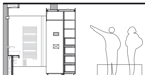
Coupe sur le meuble - séparatif :
