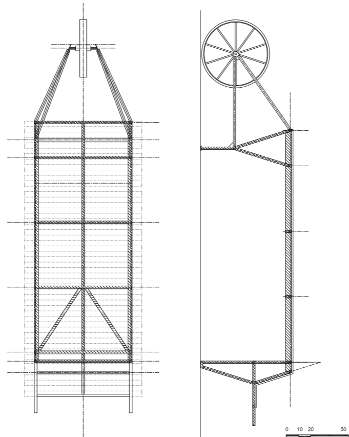
PLAN - ÉLEVATION
